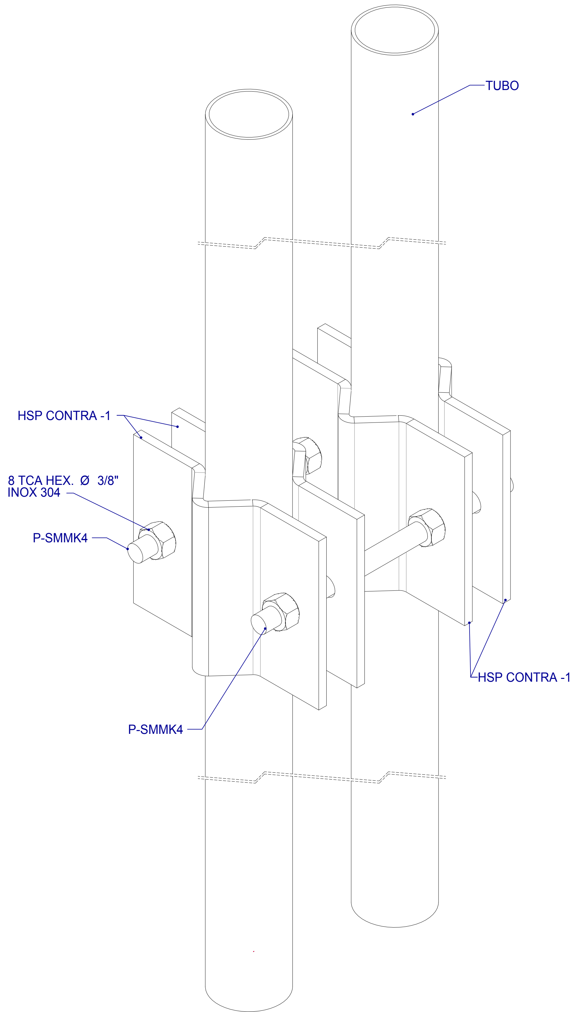
VISTA ISOMETRICA HERRAJE ADAPTADOR SMMK4
