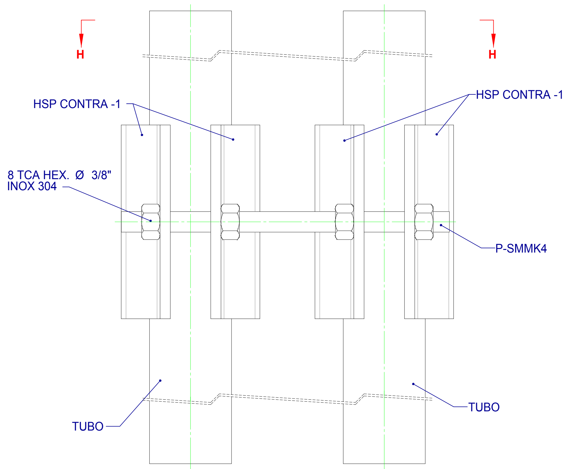
VISTA ELEVACION HERRAJE ADAPTADOR SMMK4
