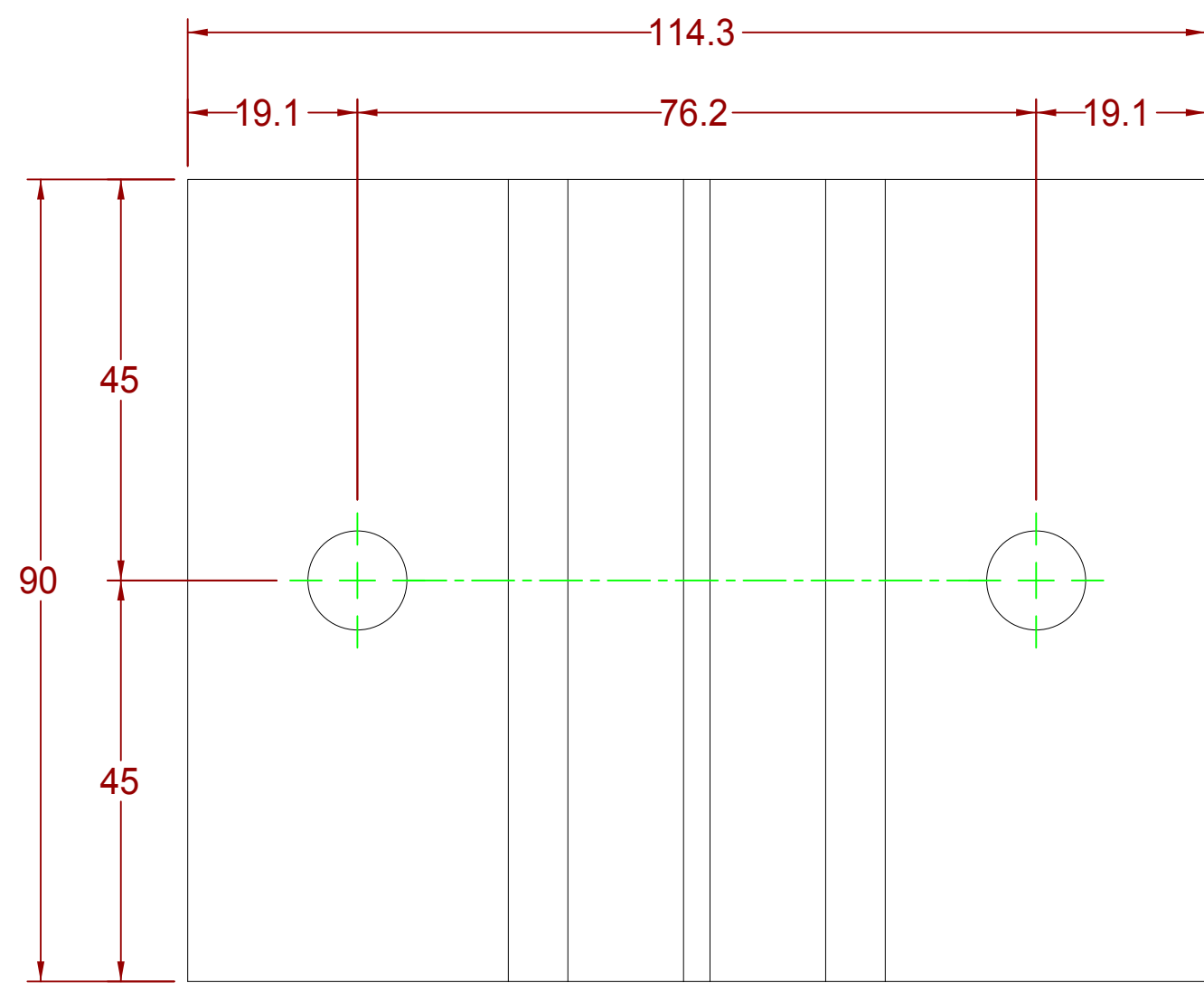
DETALLE DOBLEZ HSP CONTRA -1 (4 PZS) PLACA 3/16"
